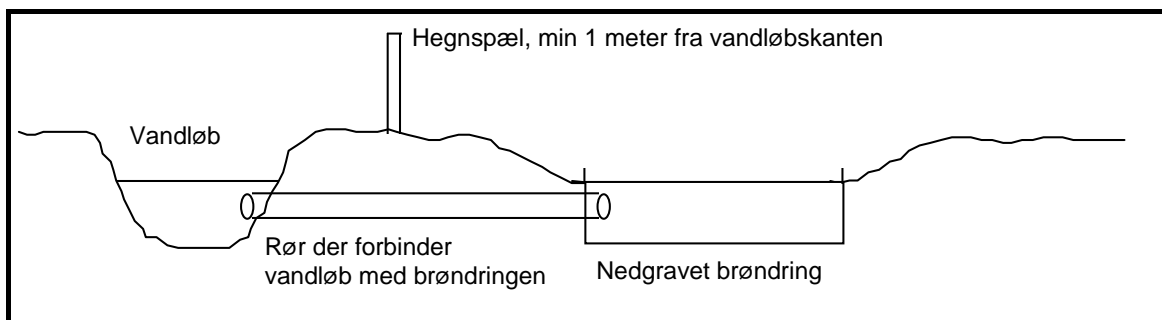
Figur 12. Skitse af nedgravet brøndring forbundet med rør til vandløbet.
